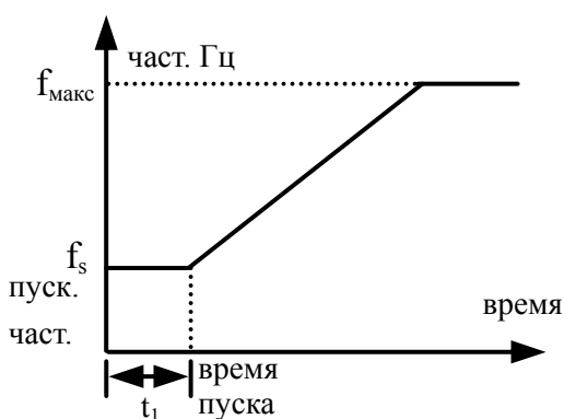
Рис.6-6 Пуск. частота и время пуска
