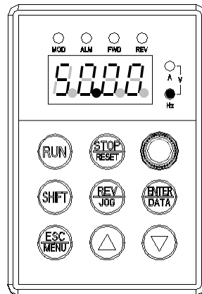
Рис.б Режим ожидания, контр. параметр для режима ожид.
