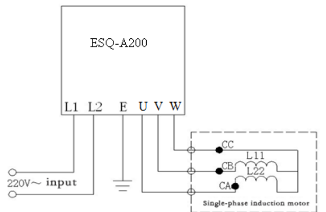
Однофазный асинхронный двигатель
